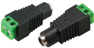
14-0315 РАЗЪЁМ питания гнездо 2.1 x 5.5 с клеммной колодкой REXANT от 12,00руб.
