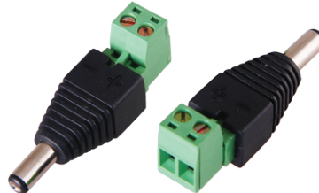
14-0314 РАЗЪЁМ питания штекер 2.1 x 5.5 с клеммной колодкой REXANT от 10,50руб.
