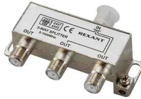
05-6002 ДЕЛИТЕЛЬ ТВ x 3 под F разъём 5-1000 МГц REXANT от 39,00руб.
