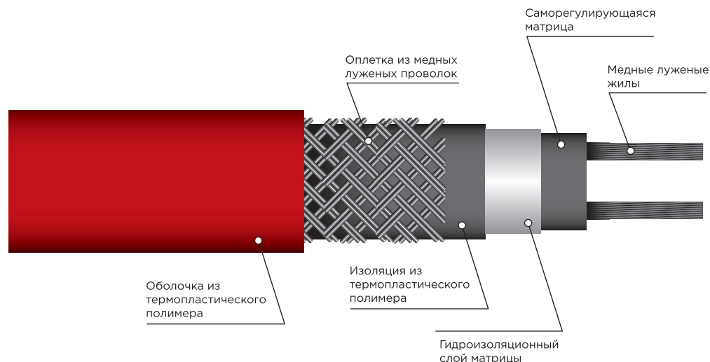
Рисунок 2.1 - Конструкция кабеля нагревательного саморегулирующегося REXANT 2.2. Принцип работы
