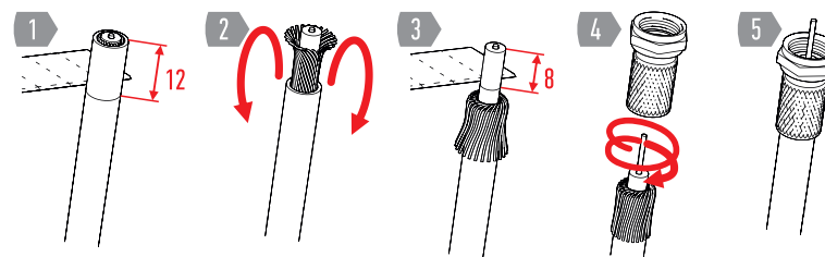
Рис. 2 Разделка кабеля
