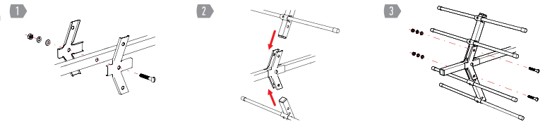
Рис. 2 Схема сборки рефлектора
