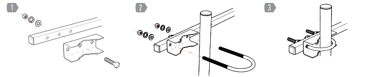
Рис. 3 Схема сборки узла крепления
