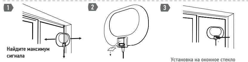
Установка на оконное стекло
